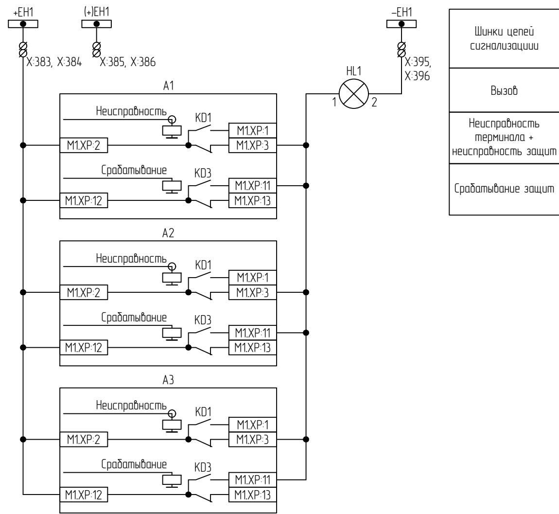
Цепи РАС
