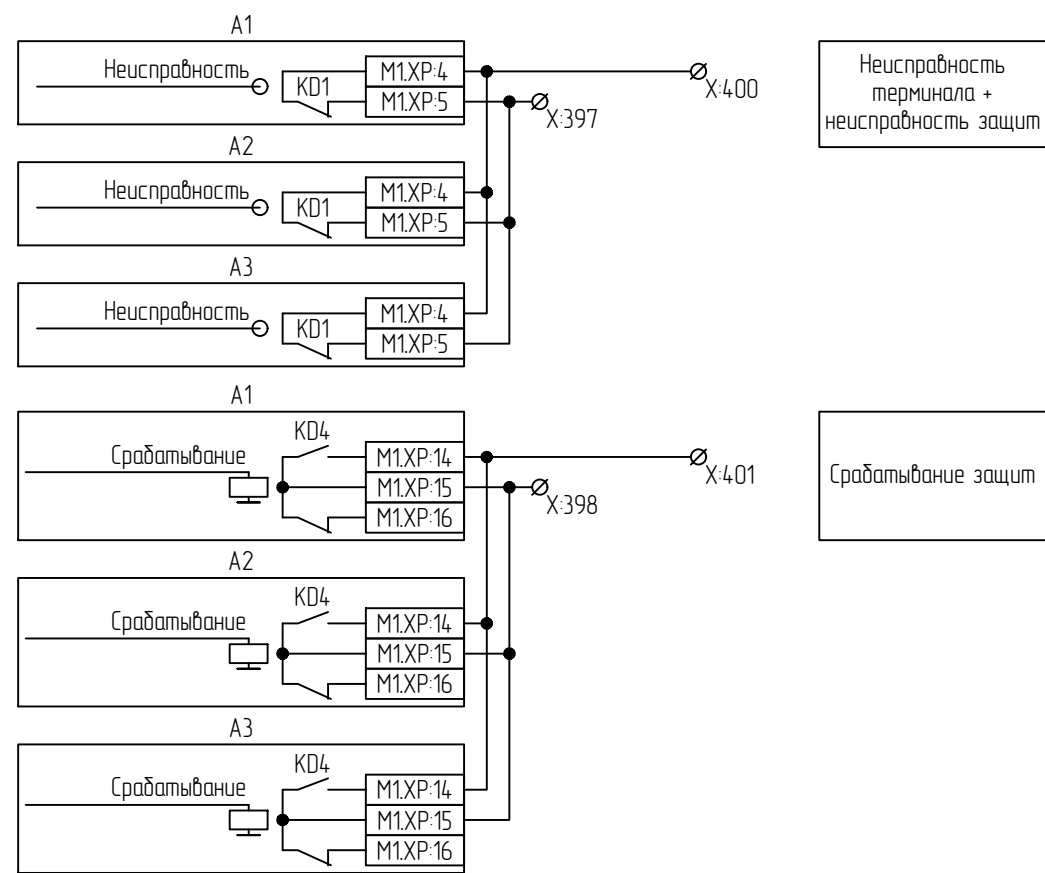
Цепи РАС
