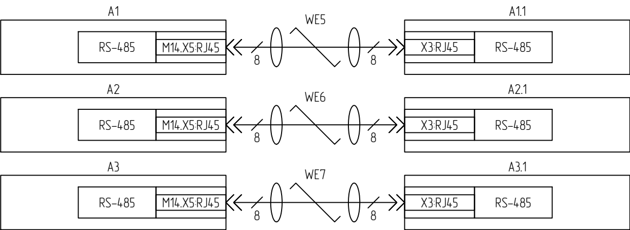
Цепи портов связи терминала
